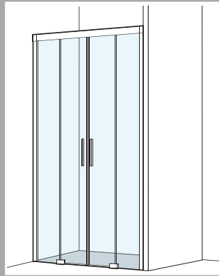
Schiebetür in Nische 4-teilig, V1-DS4N
