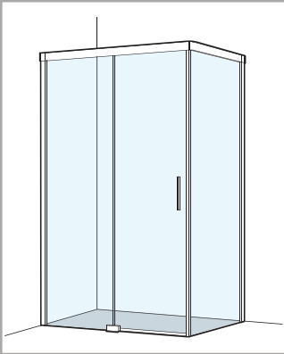
Schiebetür mit Trennwand am beweglichen Element 2-teilig, V1-DS2BTW
